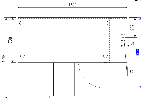
Dessus
